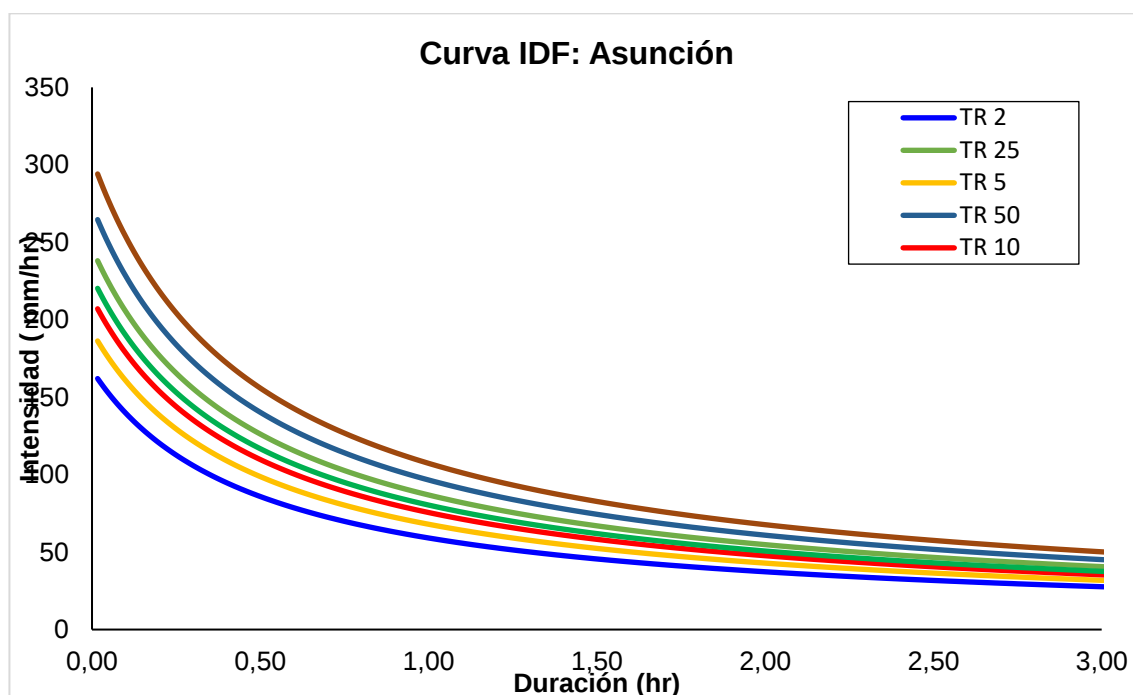
Figura 15. Curvas IDF de Asunción para diferentes tiempos de retorno.
