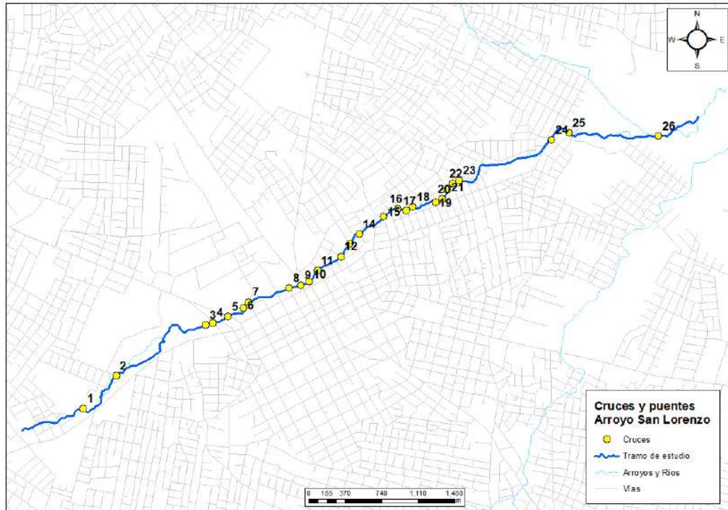
Figura 4. Tramo de estudio, con cruces - Arroyo San Lorenzo
