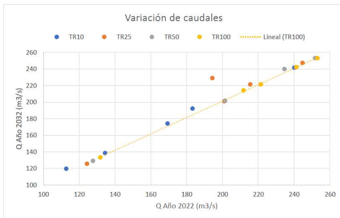
Figura 20. Variación de caudales con ponderación al 2023
