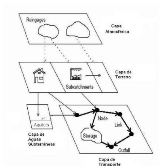
Figura 5. Modelo Conceptual del sistema de drenaje urbano
