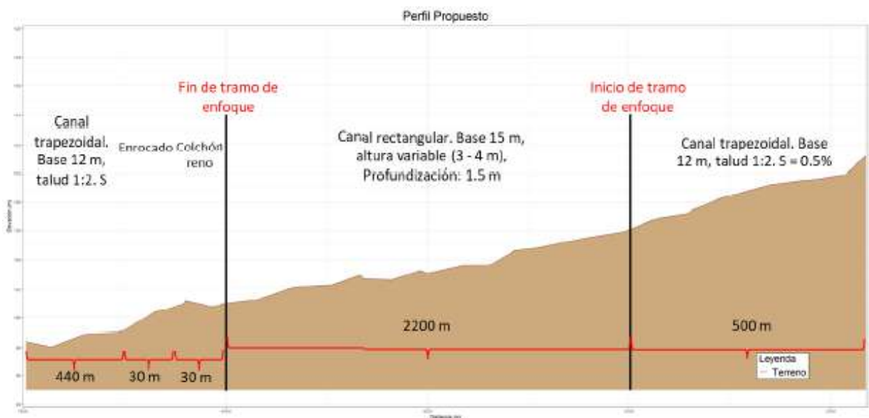
Figura 41. Esquema de propuestas de adecuación del cauce
