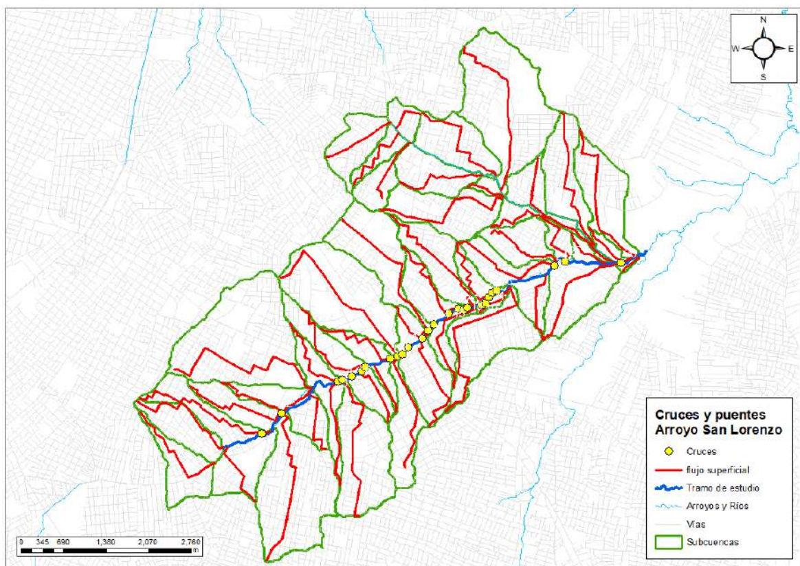
Figura 16. Red de drenaje y subcuencas para la modelación hidrológica en SWMM.
