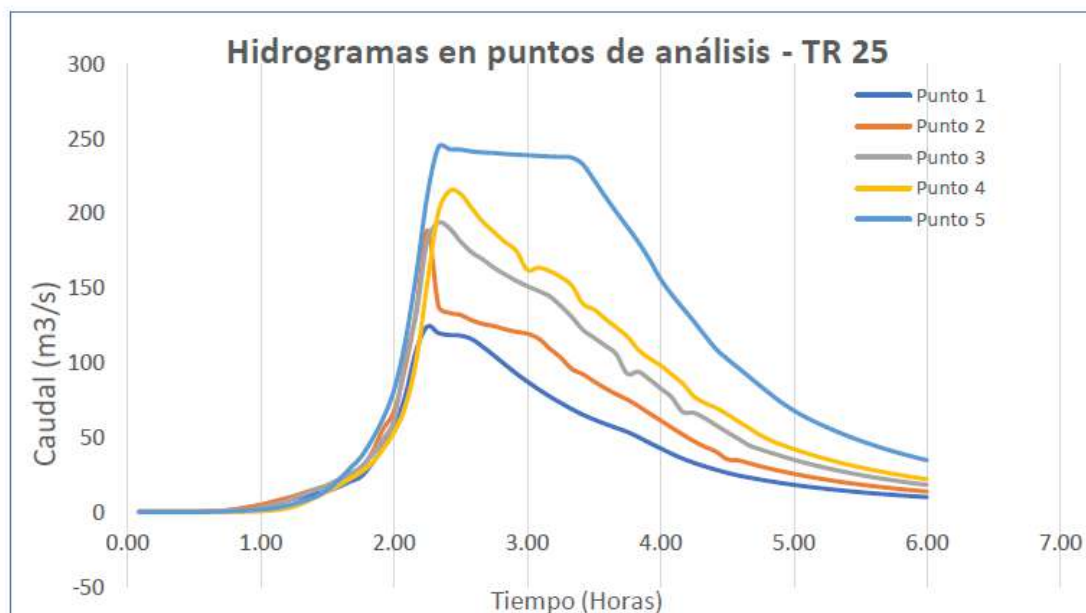
Figura 22. Hidrogramas en puntos de análisis – TR25
