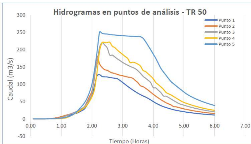
Figura 23. Hidrogramas en puntos de análisis – TR50
