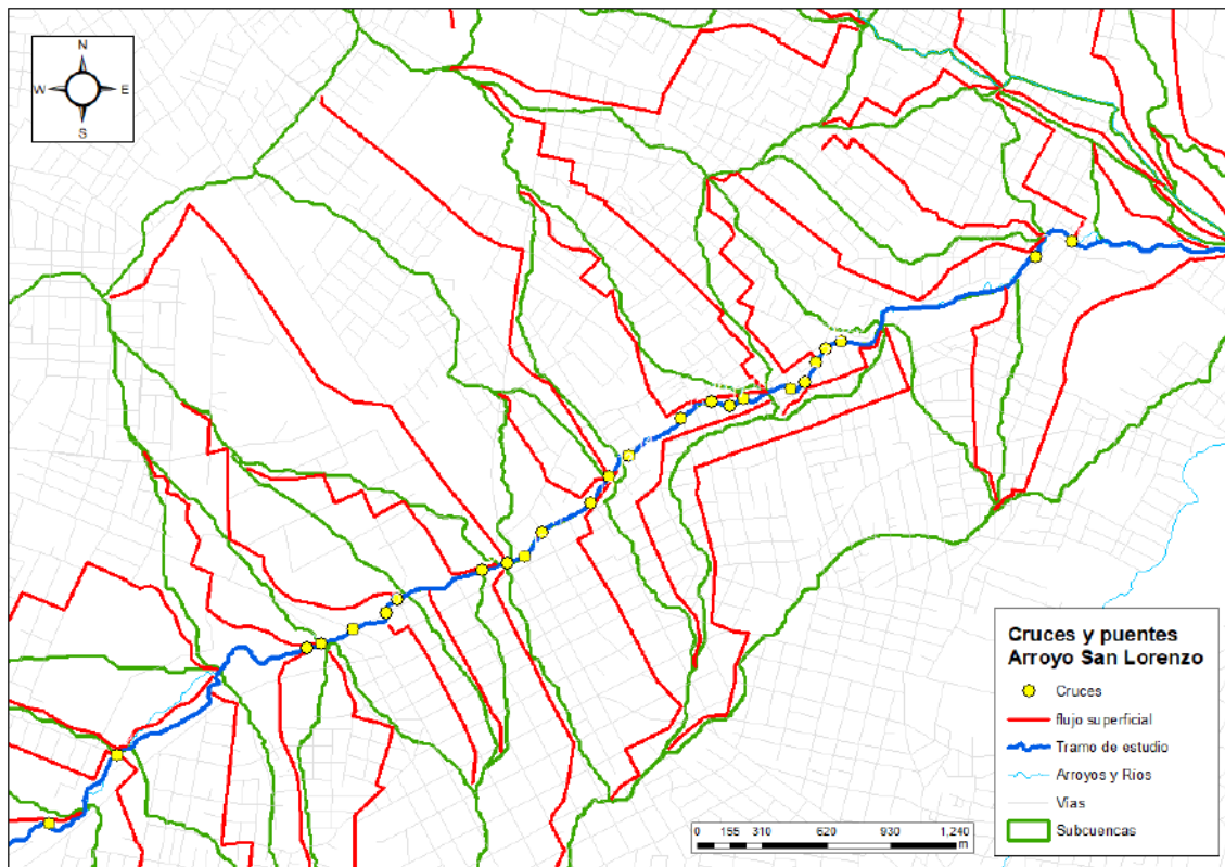
Figura 17. Red de drenaje y subcuencas para la modelación hidrológica en SWMM - zoom.
