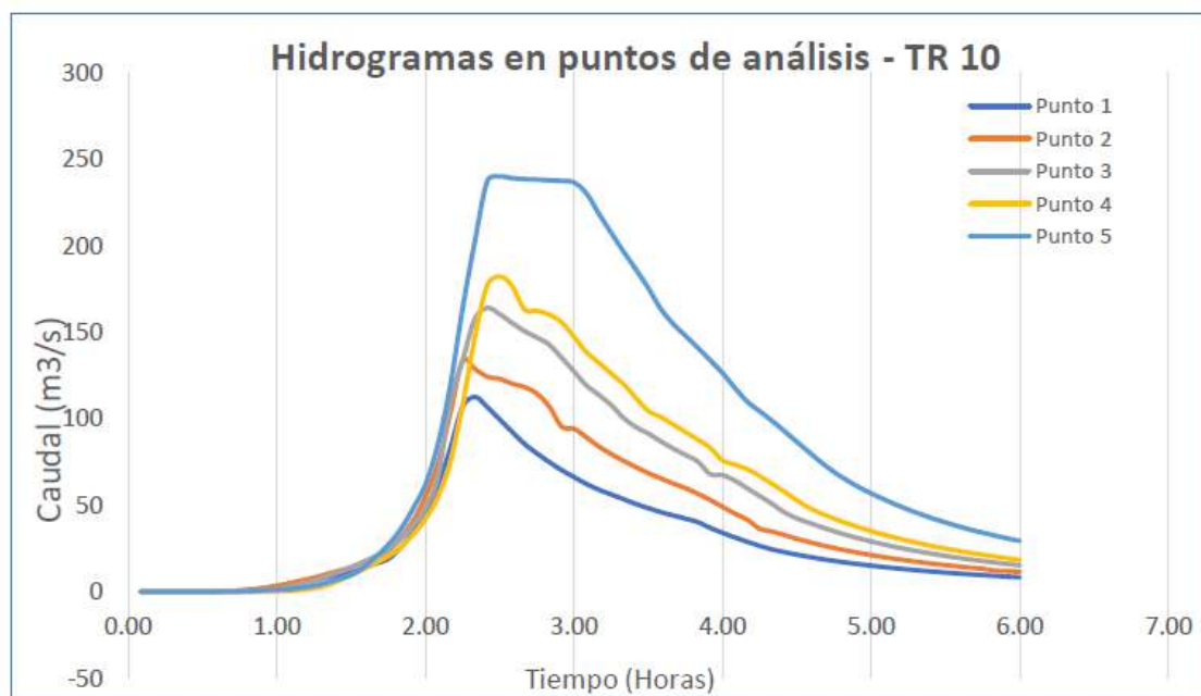
Figura 21. Hidrogramas en puntos de análisis – TR10
