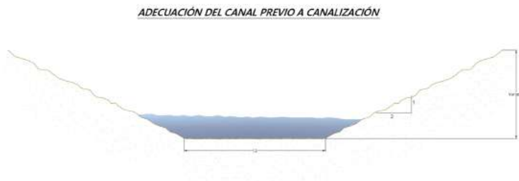
Figura 34. Canal trapezoidal recomendado para tramos de adecuación
