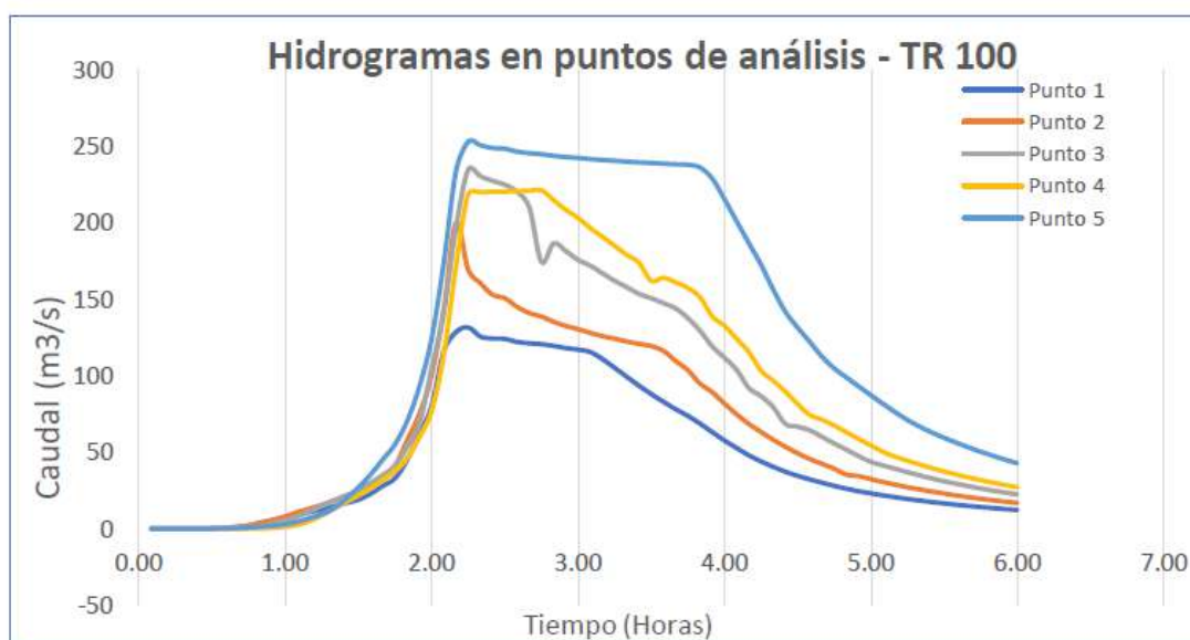
Figura 24. Hidrogramas en puntos de análisis – TR100
