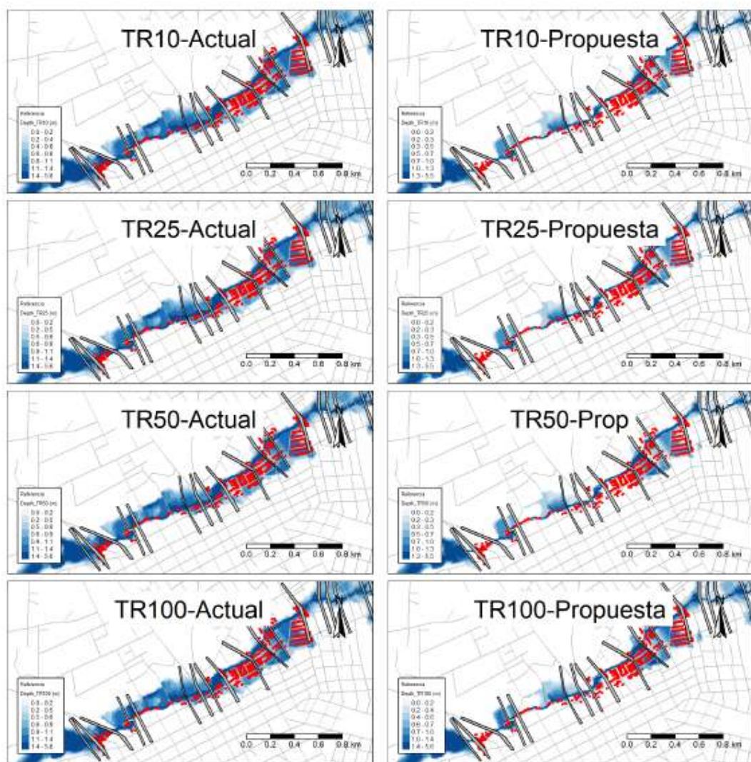
Figura 36. Comparación de superficie inundada con las propuestas implementadas
