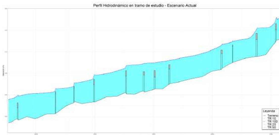
Figura 31. Perfil hidrodinámico para el tramo de enfoque – Escenario Actual
