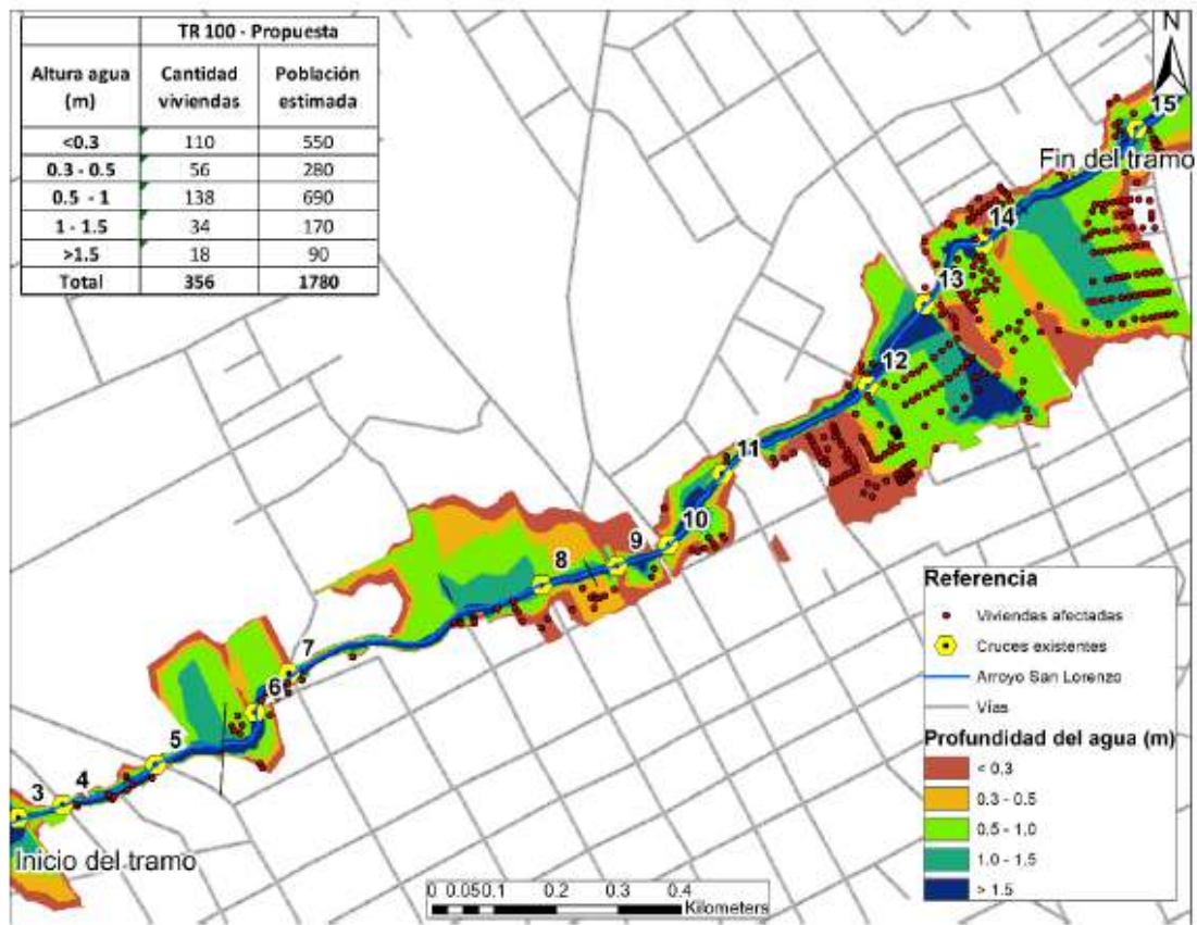
Figura 40. Riesgos asociados a inundación – Escenario propuesto
