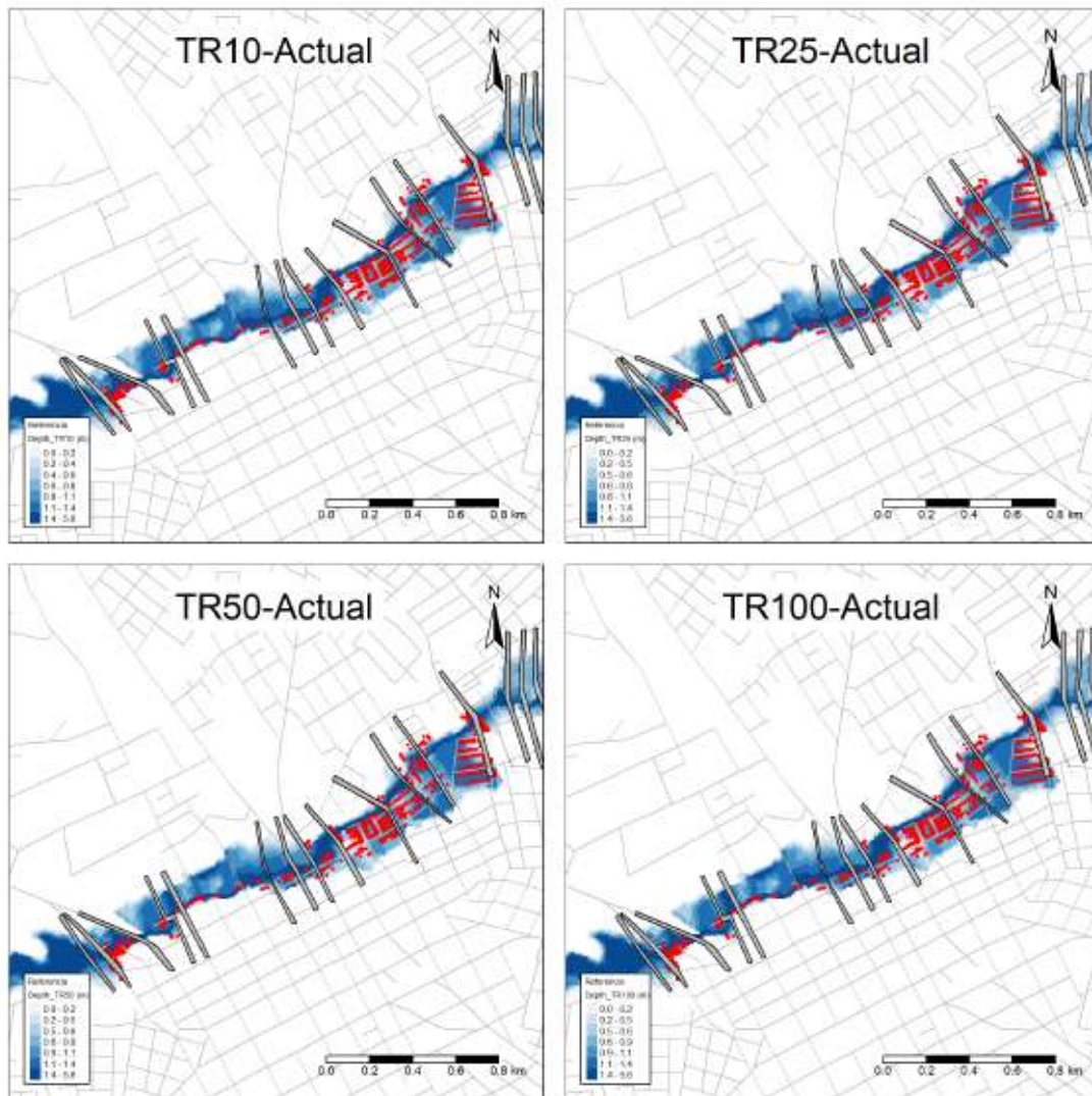
Figura 29. Superficie inundada para el escenario actual – Tramo de enfoque
