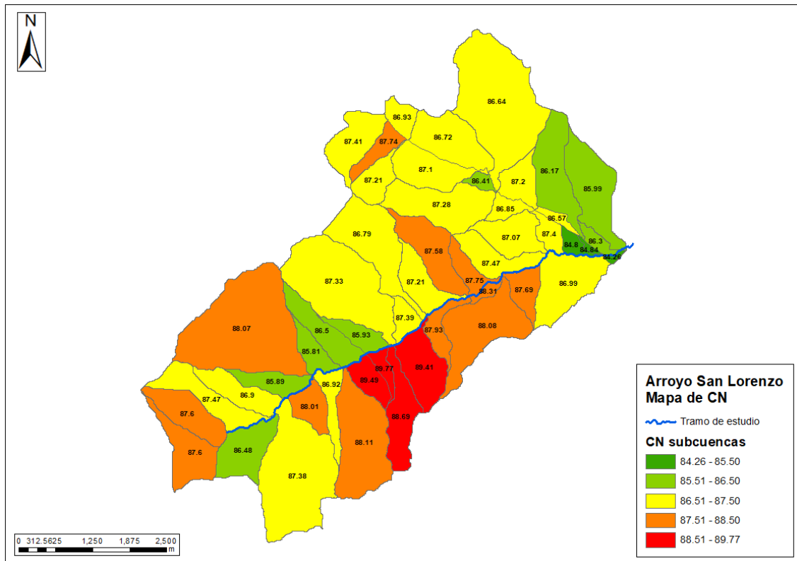
Figura 14. Numero de curvas (CN) por cuenca
