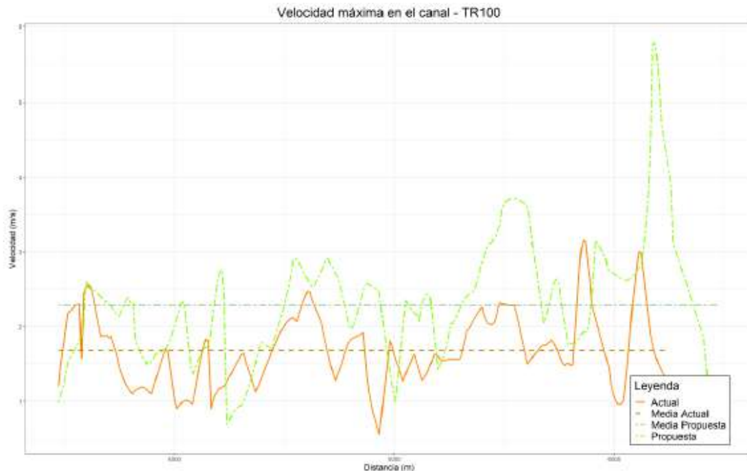
Figura 38. Velocidad máxima en el canal para el tramo de estudio
