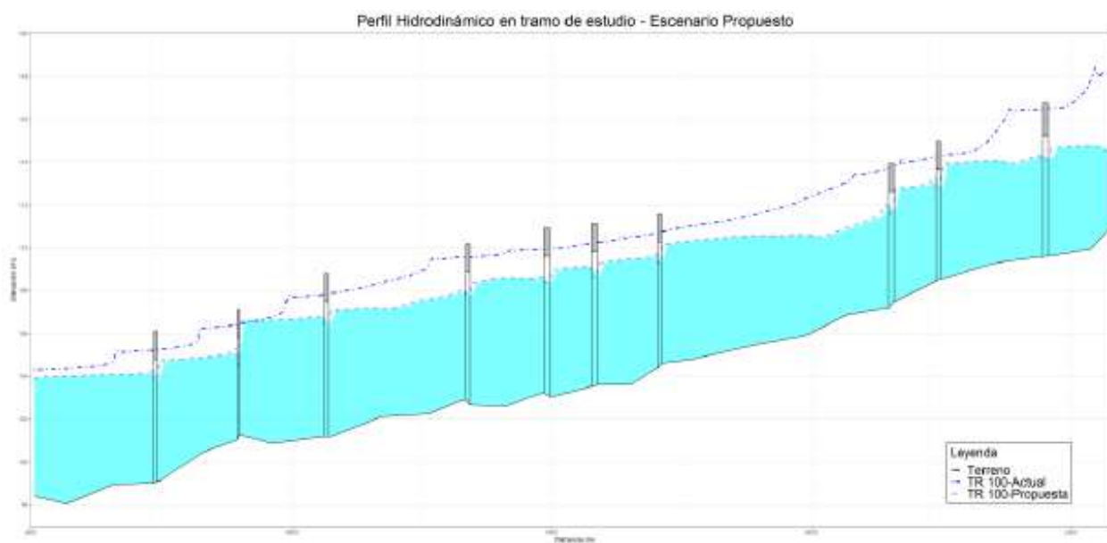
Figura 39. Perfil hidrodinámico para el tramo de enfoque – Escenario propuesto
