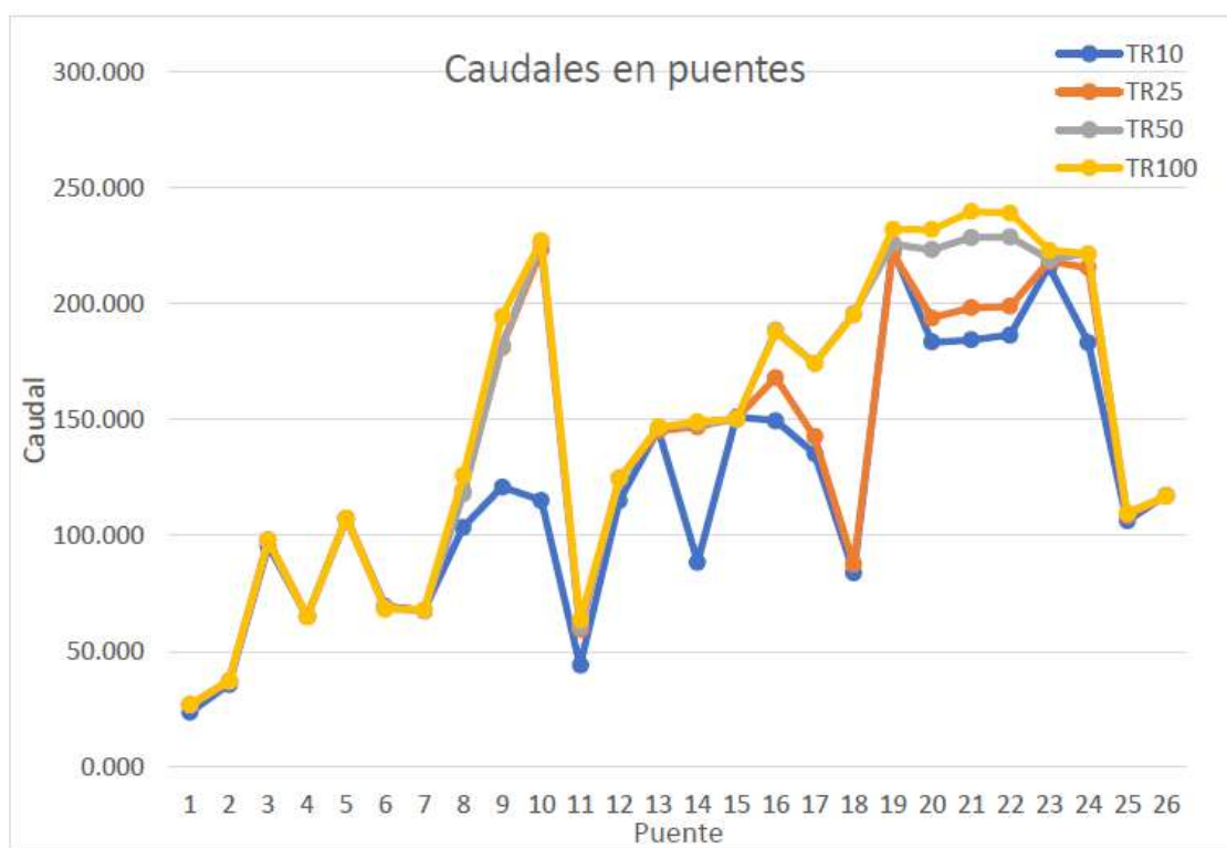
Figura 25. Comparación de caudales en los puentes para distintos TR
