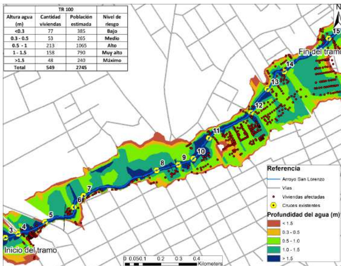
Figura 32. Riesgos asociados a inundación – Escenario actual
