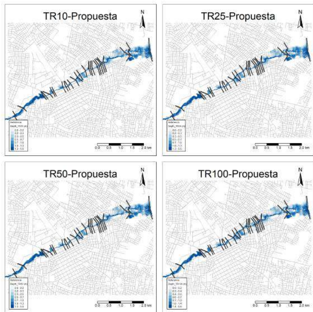
Figura 35. Superficie inundada para el escenario propuesto – Tramo completo
