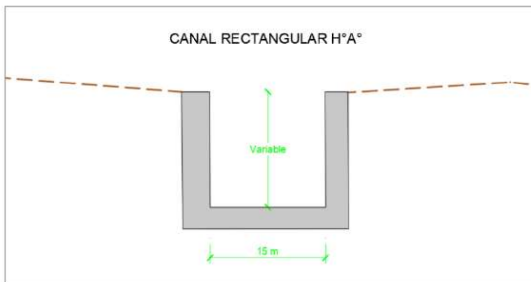
Figura 33. Canal de H°A° recomendado
