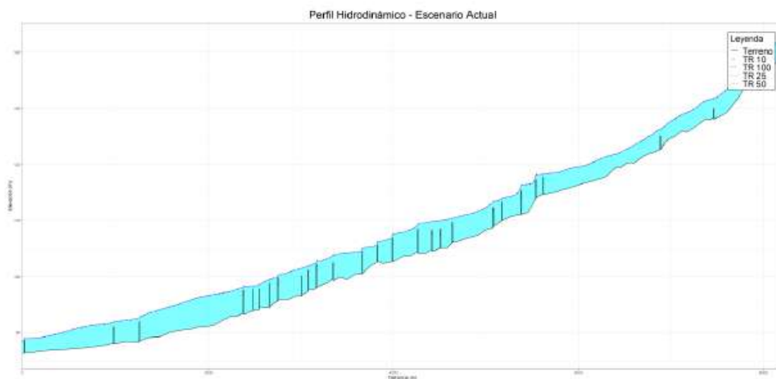
Figura 30. Perfil hidrodinámico para el tramo general – Escenario Actual
