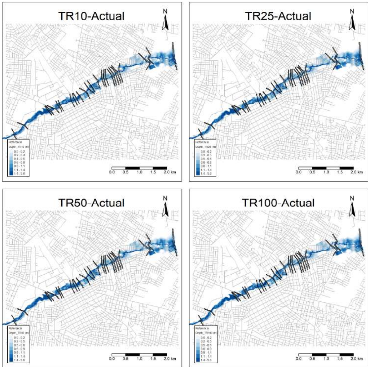
Figura 28. Superficie inundada para el escenario actual – Tramo completo
