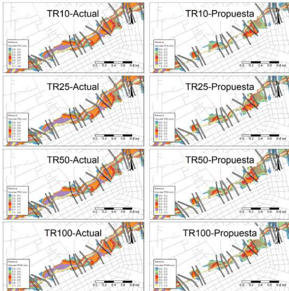
Figura 37. Comparación de velocidades máximas obtenidas con las medidas propuestas
