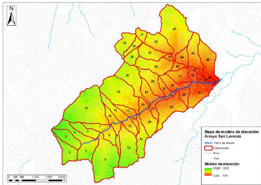
Figura 8. Cuencas delimitadas sobre modelo de elevación del terreno
